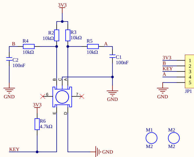
旋转编码器
