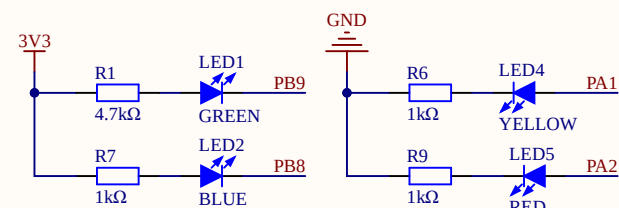
控制电路
