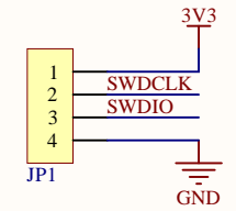
SW调试
