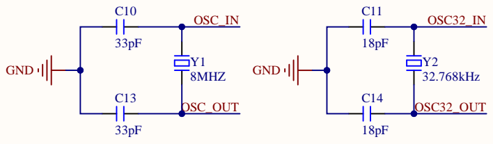
晶振电路
