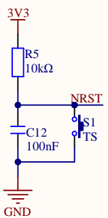
复位电路
