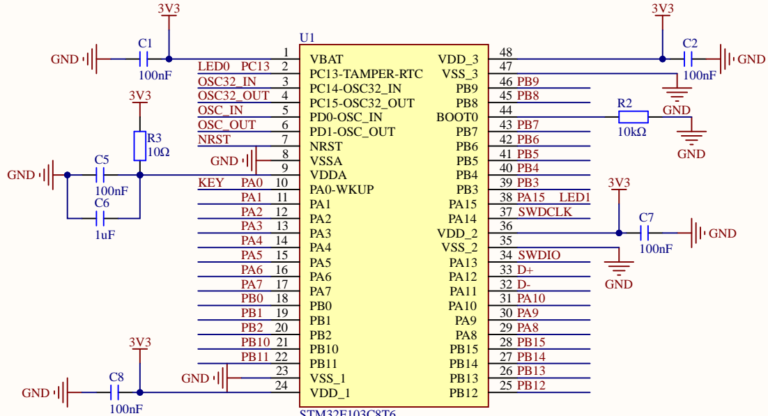
主控芯片
