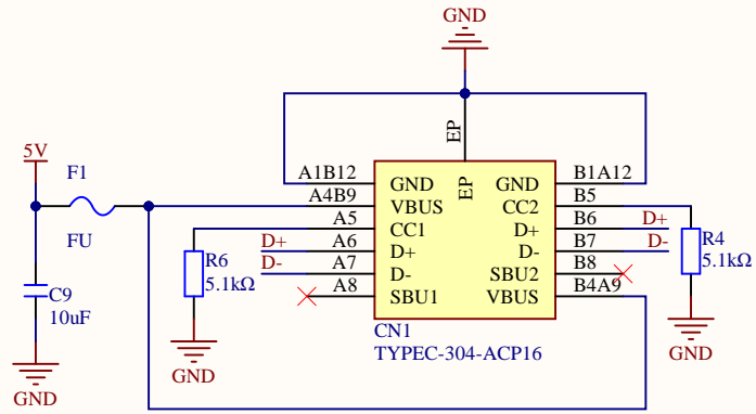
TYPEC接口
